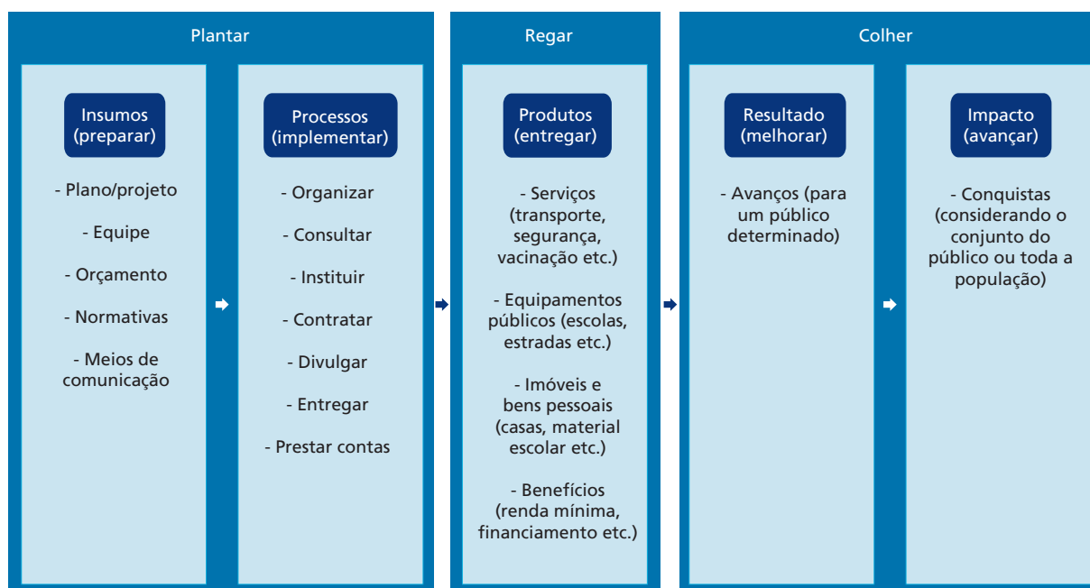
FIGURA 10 Modelo lógico
